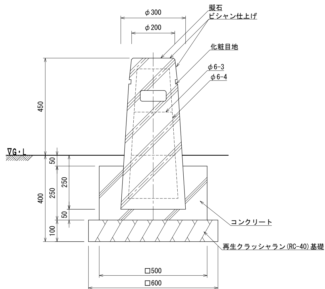
断面図
