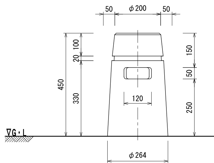
立面図
