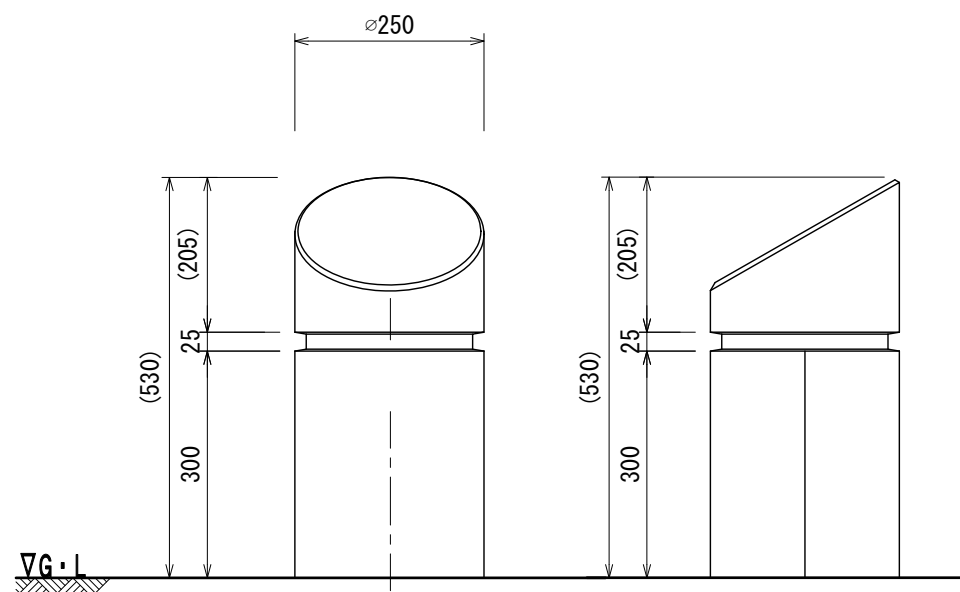
立面図
