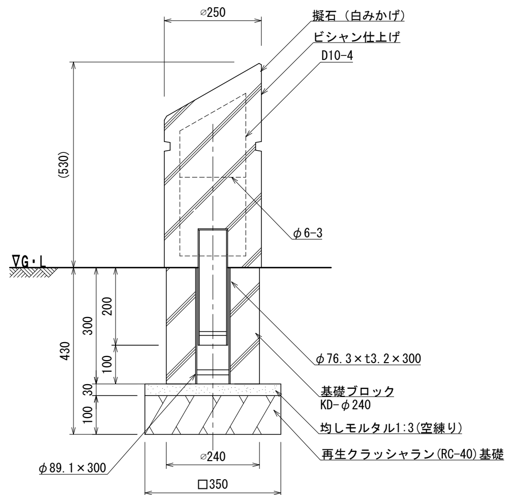
断面図
