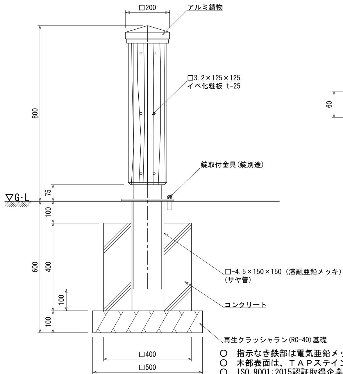
断面図 S=1:5
