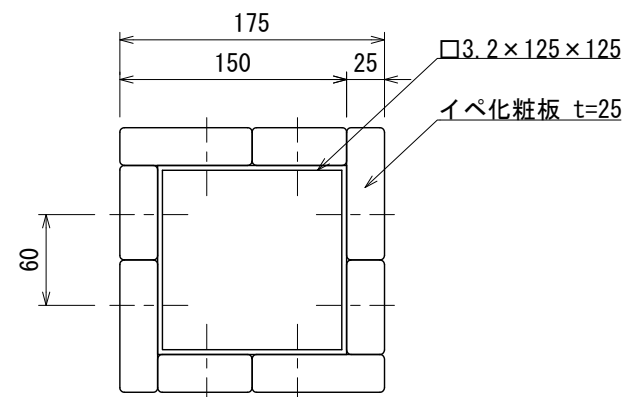
断面図 S=1:5
