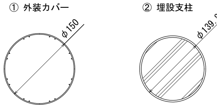
主要部材断面図 (S=1:5)
