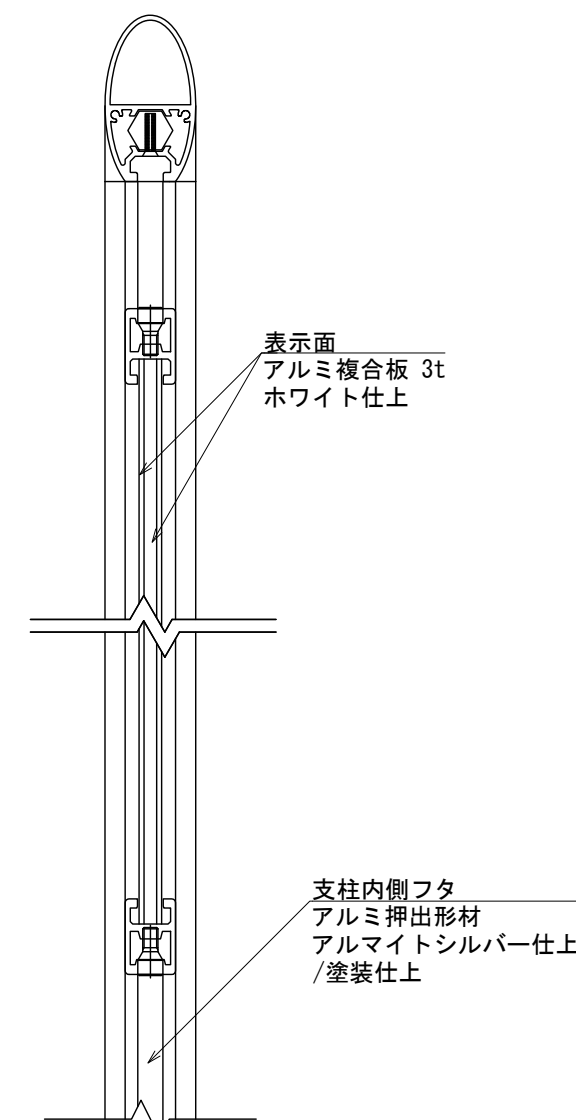
【側面図 S=1:3】
