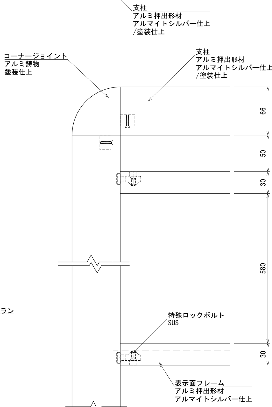
【正面図 S=1:3】
