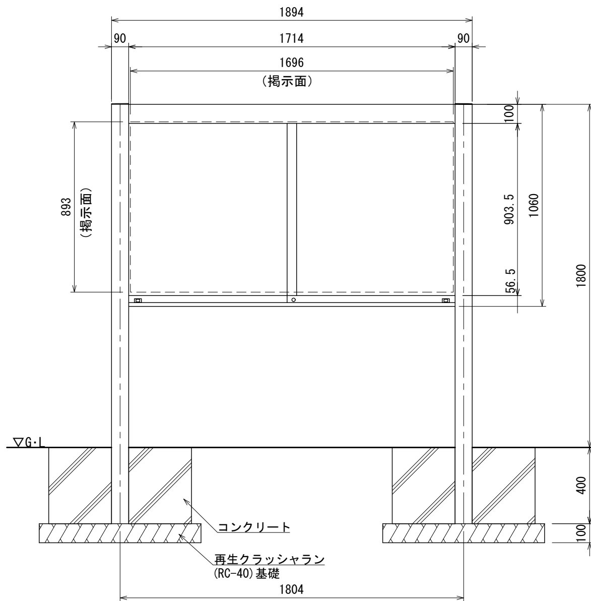
【正面図】
