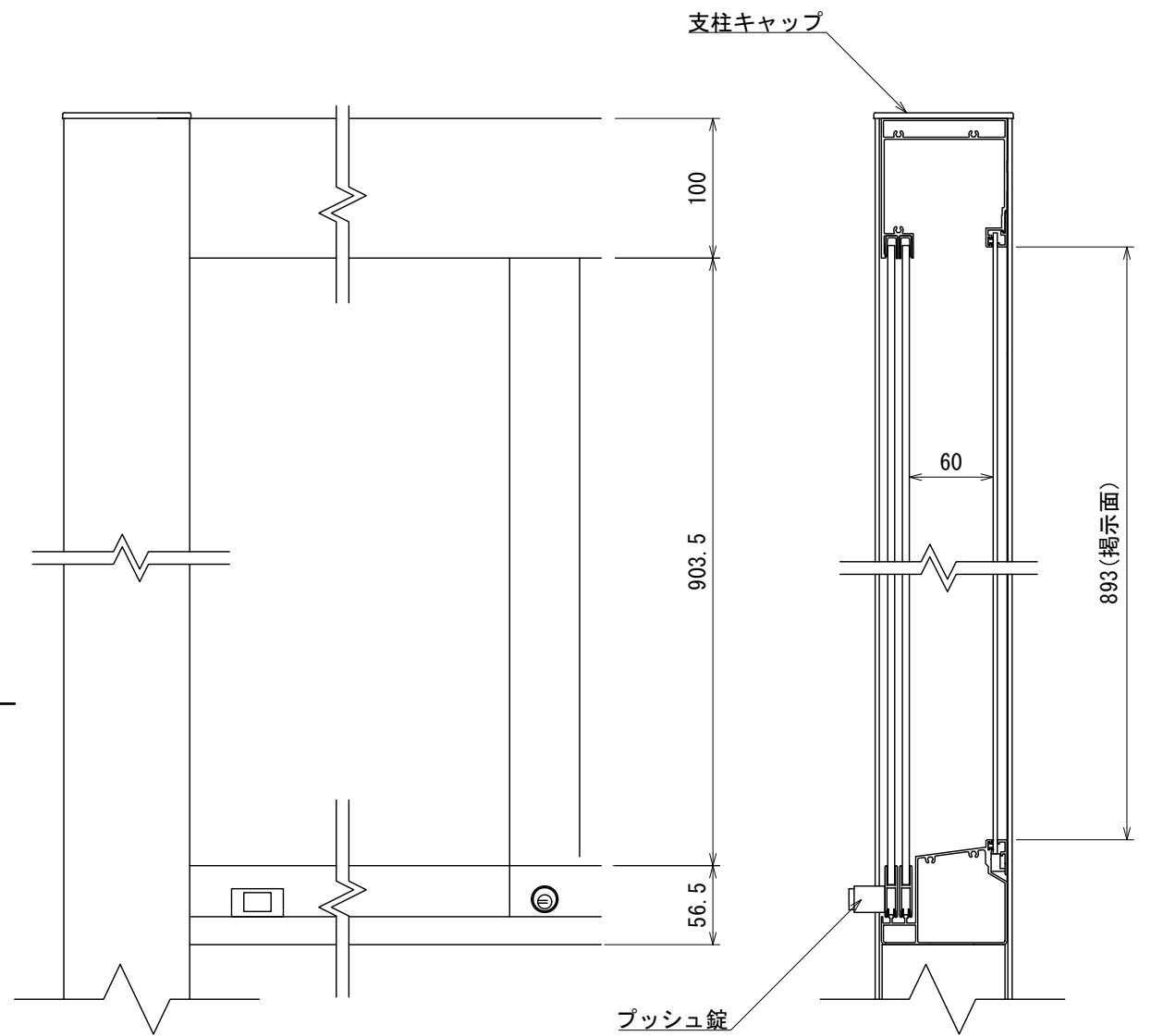
【正面図 S=1:5】
