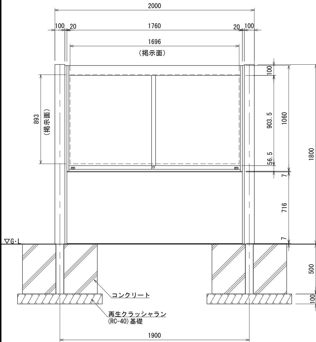
【正面図】
