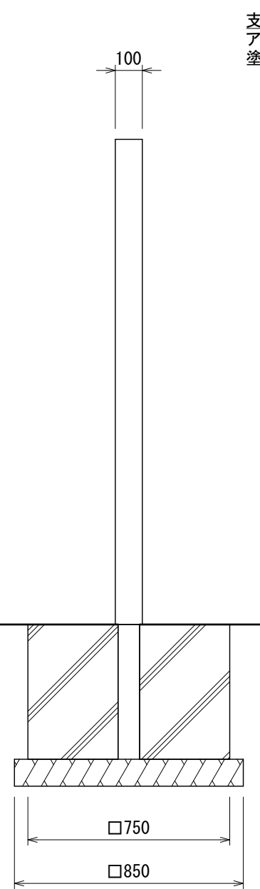
【側面図】
