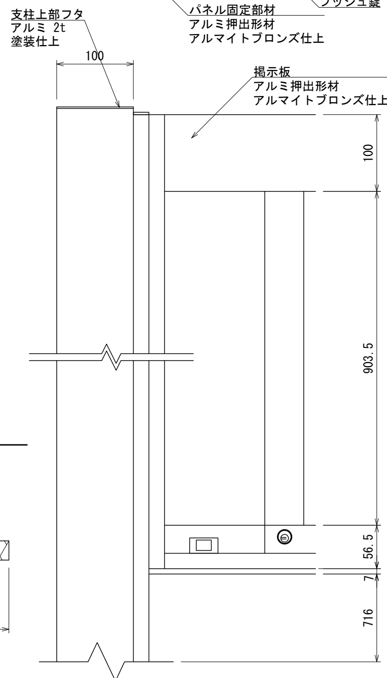
【正面図 S=1:5】
