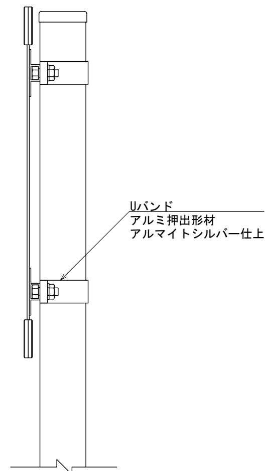
【側面図 S=1:5】
