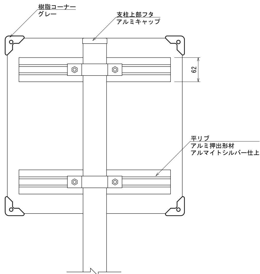
【背面図 S=1:5】
