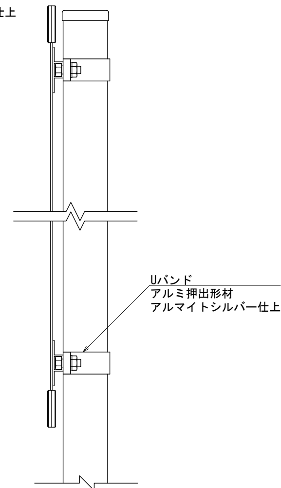
【側面図 S=1:5】
