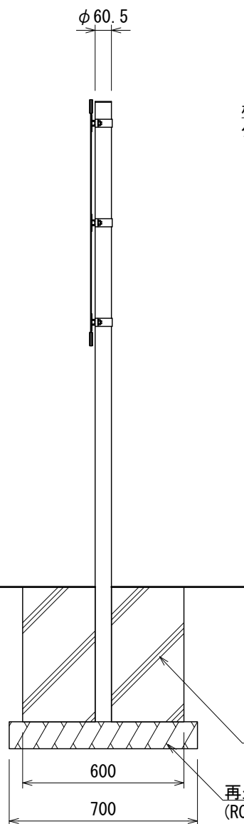
【側面図】
