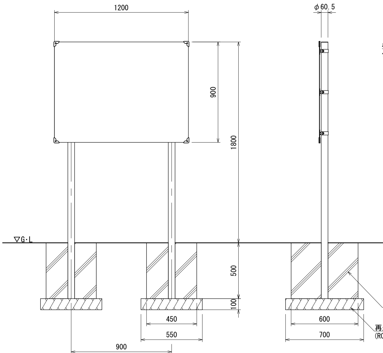
【正面図】
