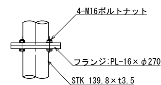
フランジ部取付詳細図 S=1:10 (A3 S=1:20)
