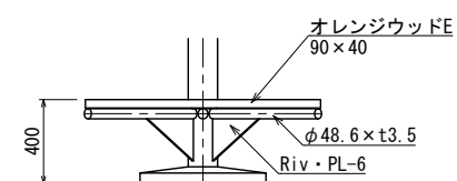
ベンチ詳細図 S=1:20 (A3 S=1:40)
