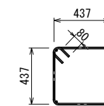
② フープ筋(TOP): 2-D13
