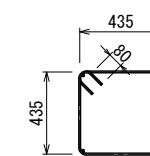
③ フープ筋: 4-D10
