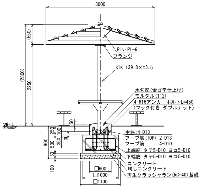
立面図
