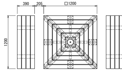
テーブルセット配置図 S=1:20 (A3 S=1:40)
