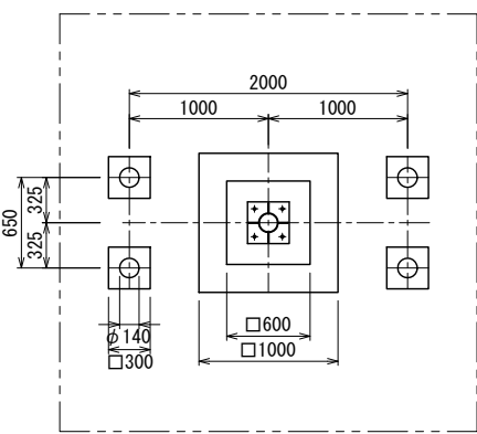
基礎伏図
