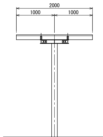
側面図
