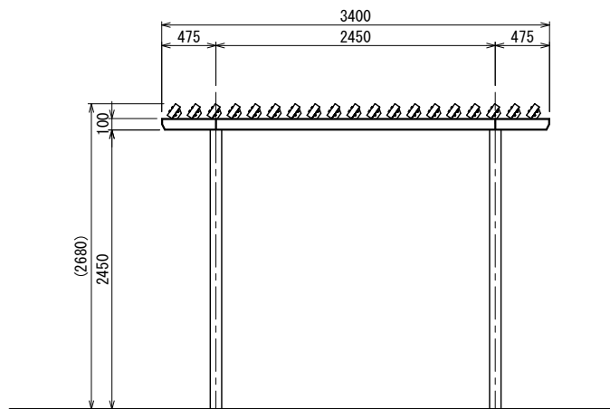
立面図
