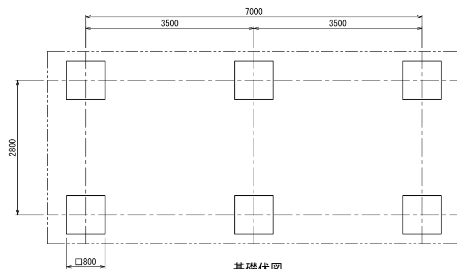
基礎伏図
