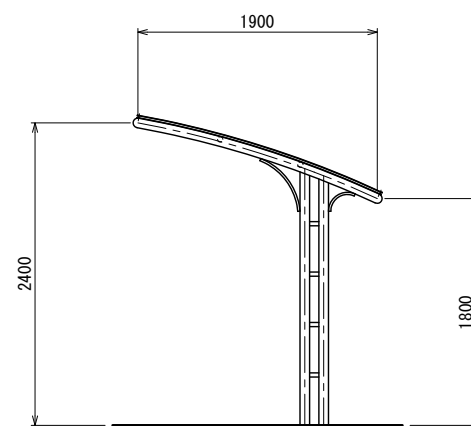
側面図
