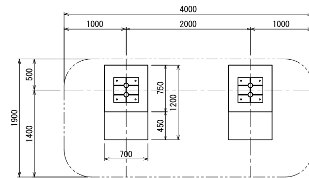
基礎伏図
