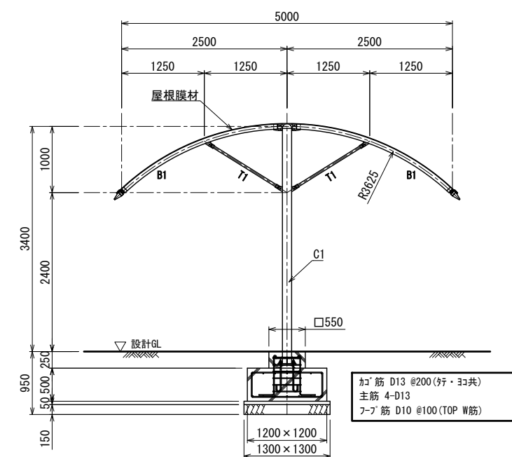
(a-a) 断面図
