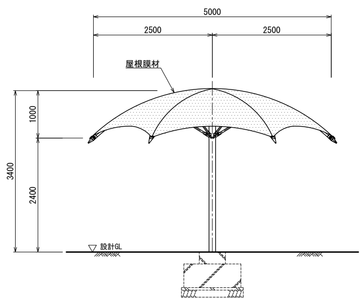
立面図
