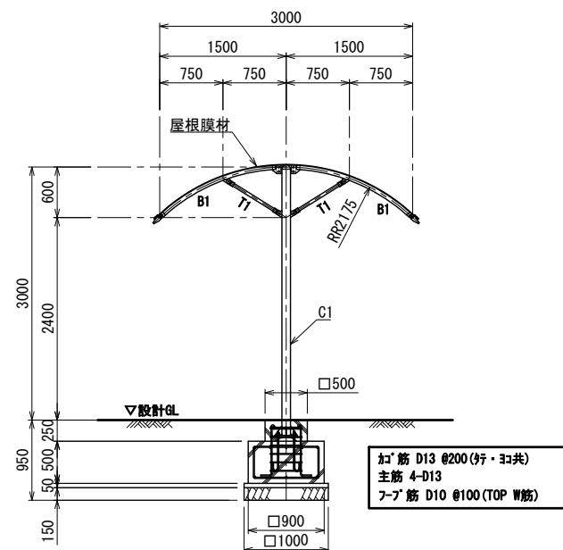
(a)-(a) 断面図
