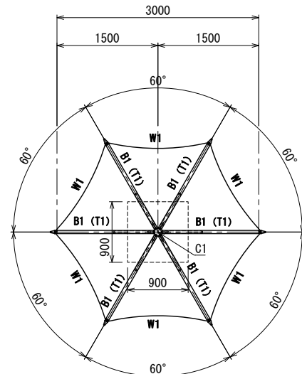
小屋伏図
