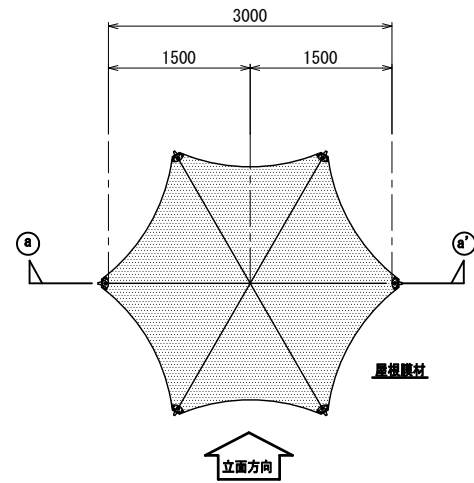
屋根膜材
