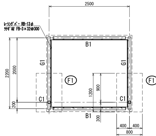
小屋伏図
