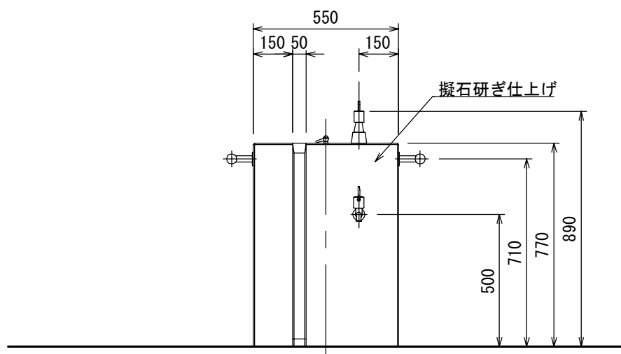
正面図
