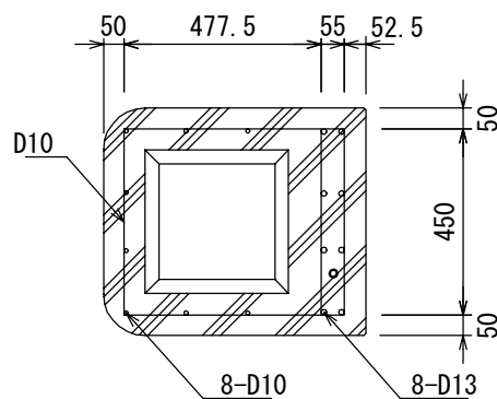
C-C断面図
