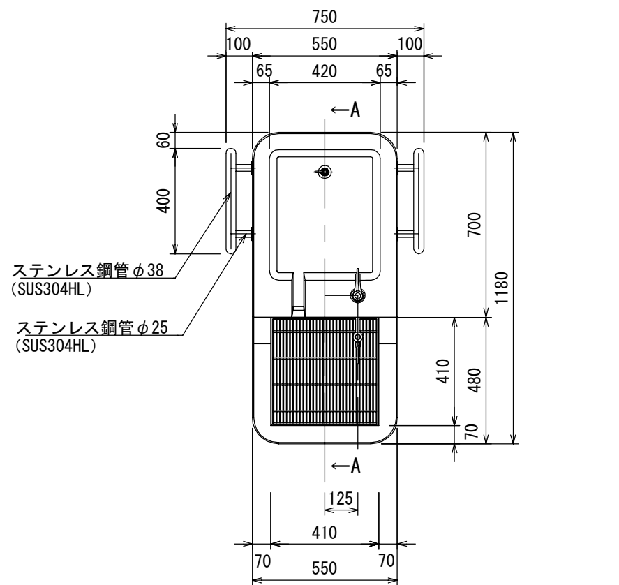
平面図
