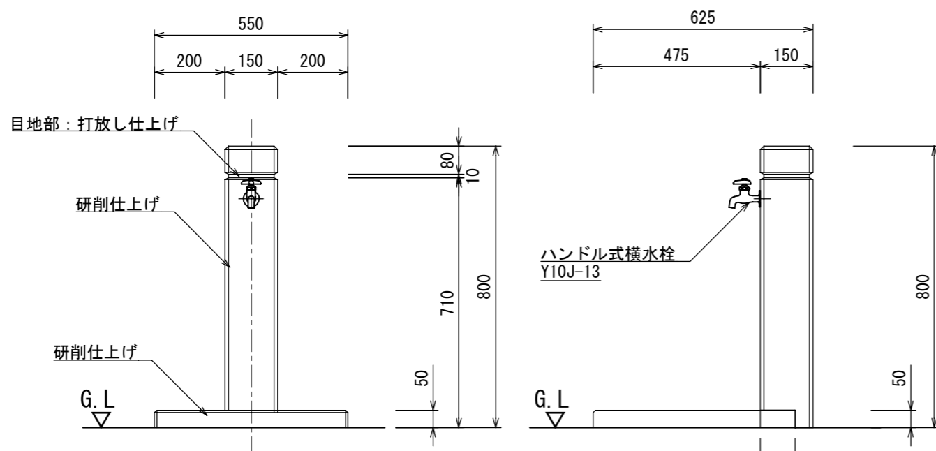
立面図
