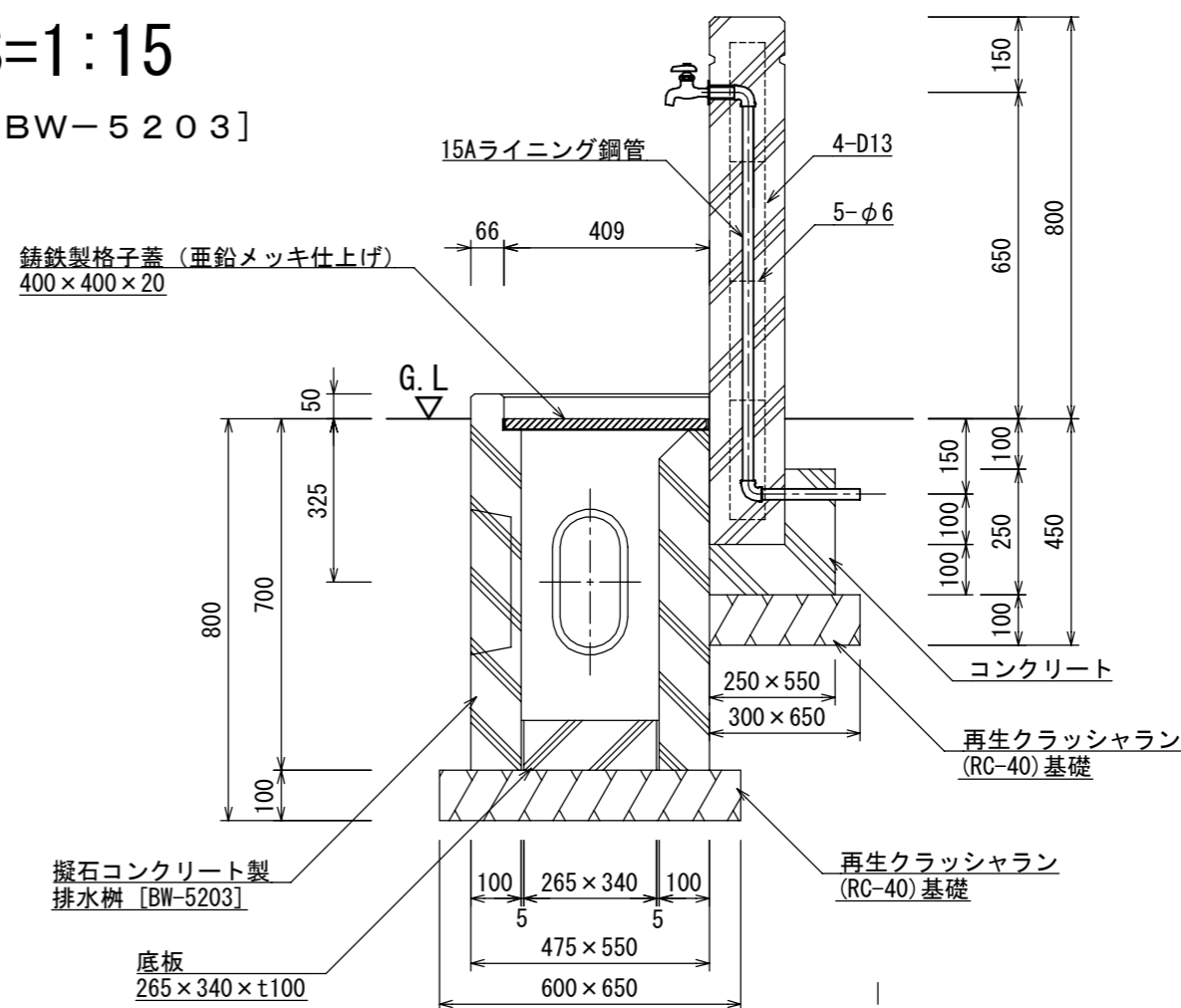
A-A断面図
