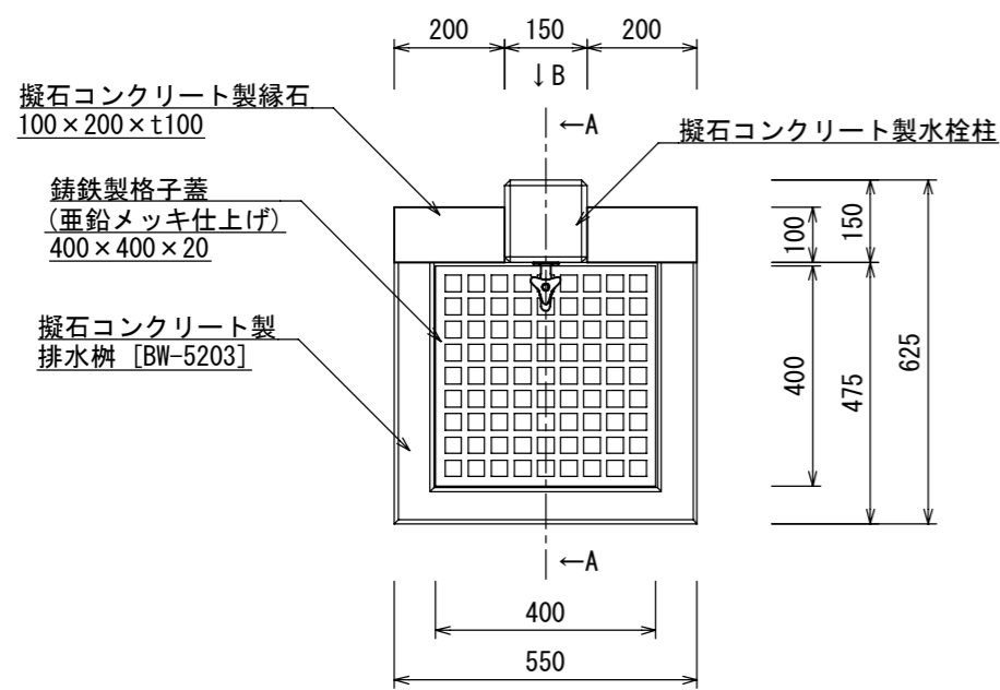
平面図
