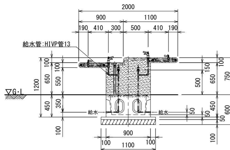
背面図
