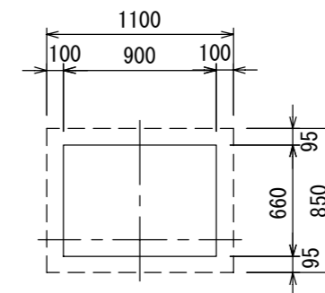
基礎伏図
