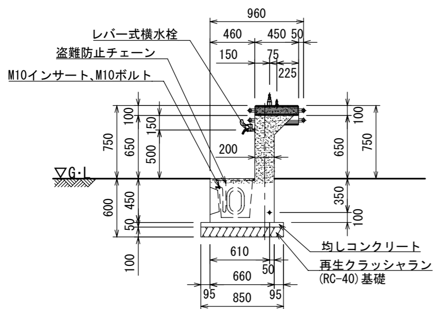
左側面図
