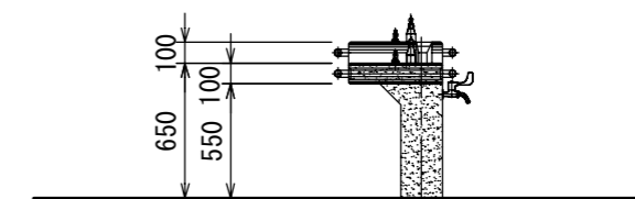
右側面図
