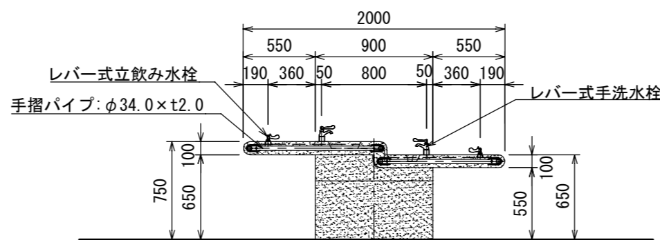
正面図
