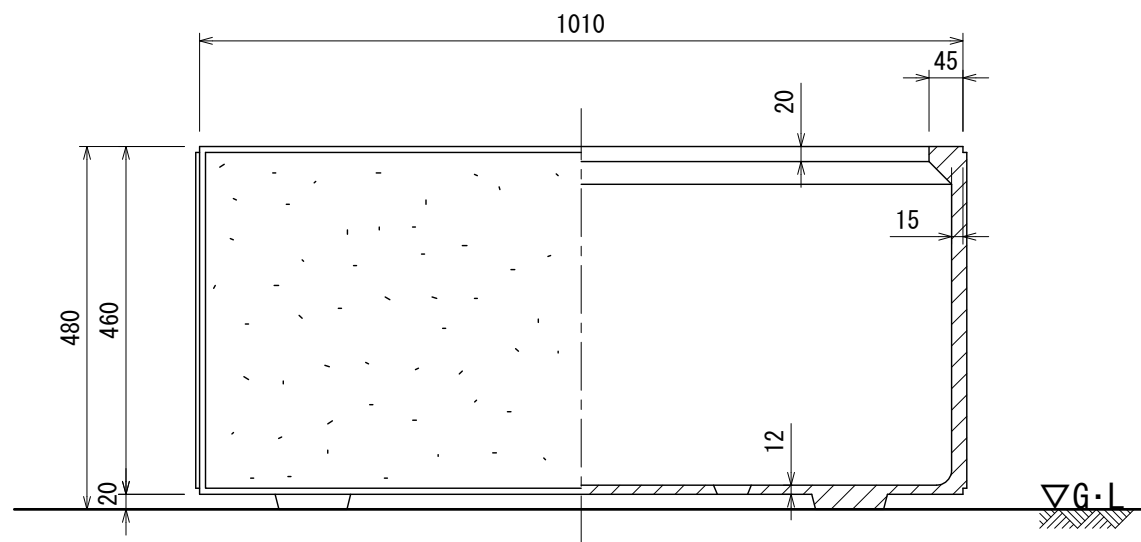
立・断面図
