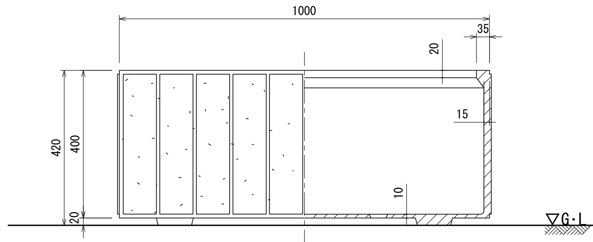
立・断面図
