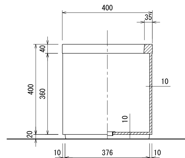
側・断面図
