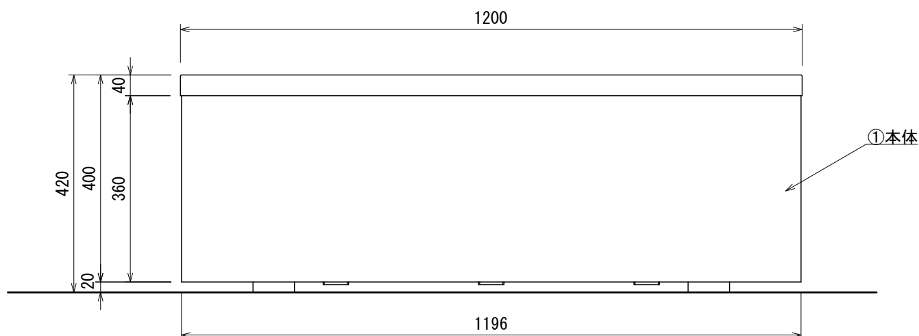
正面図
