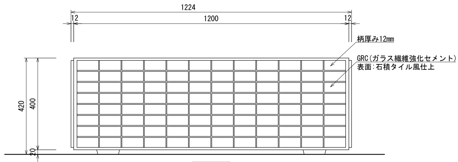
正面図
