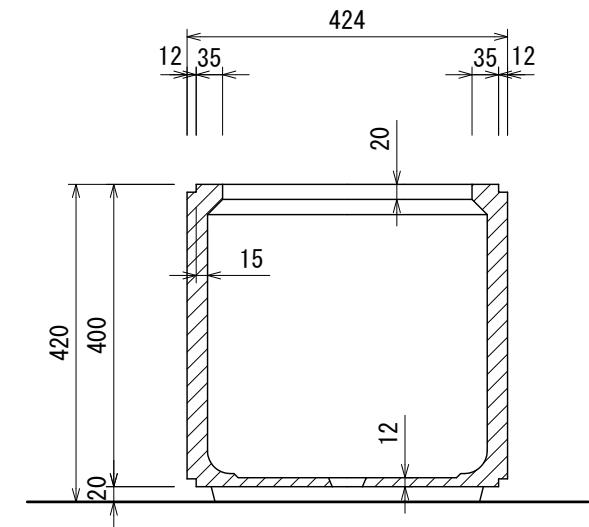
断面図
