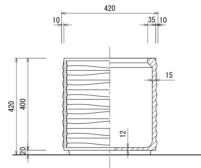
側面図・断面図
