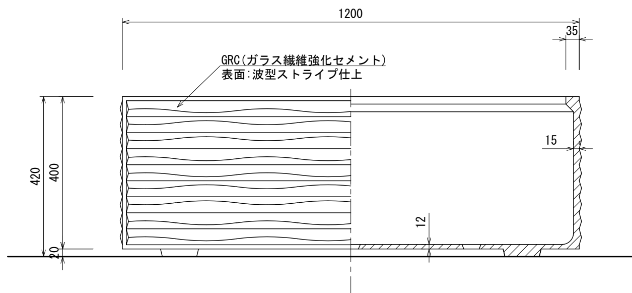
正面図・断面図
