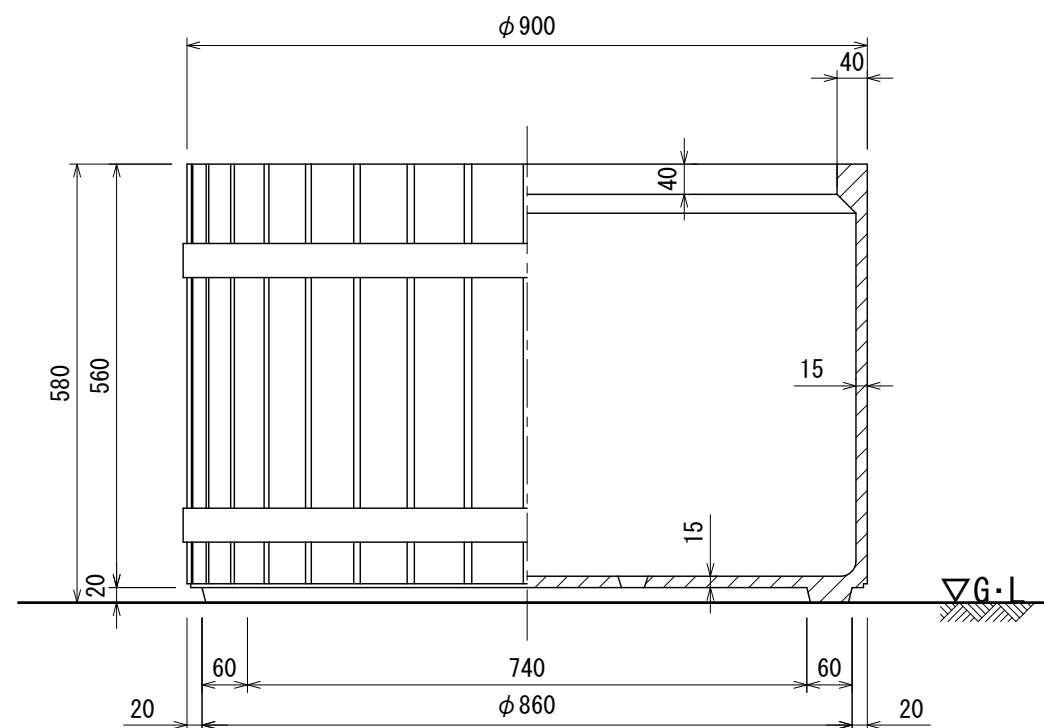
立・断面図
