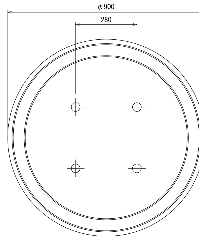
底面図
