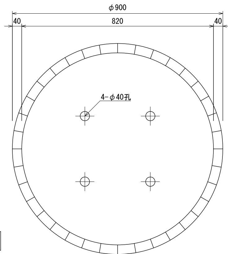
平面図
