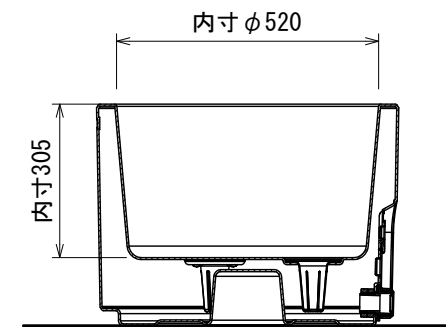
B-B' 断面図
