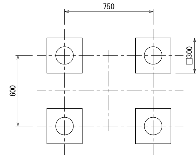
基礎伏図
