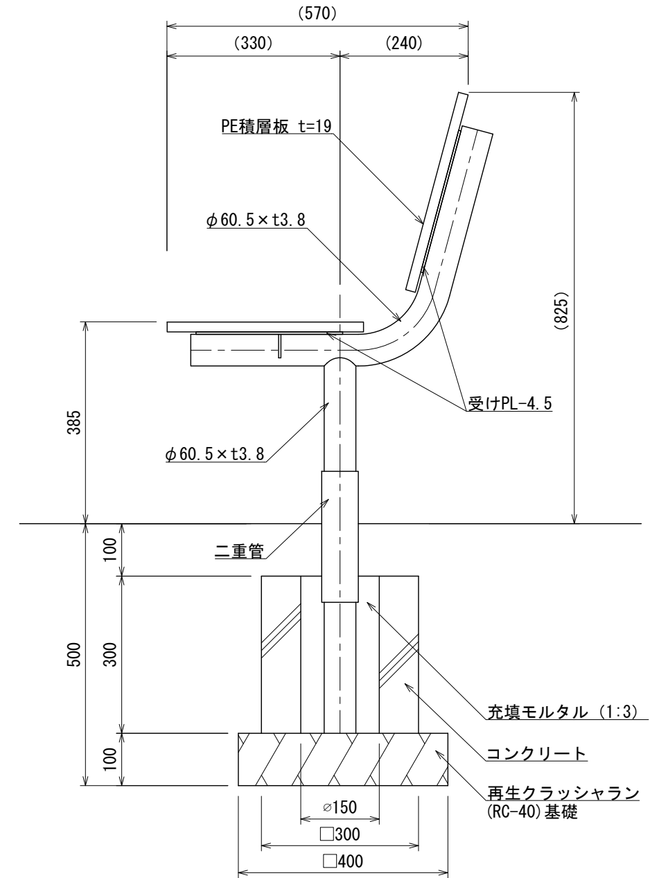
断面図
