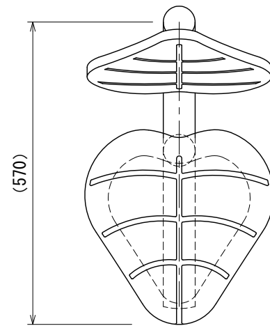
平面図
