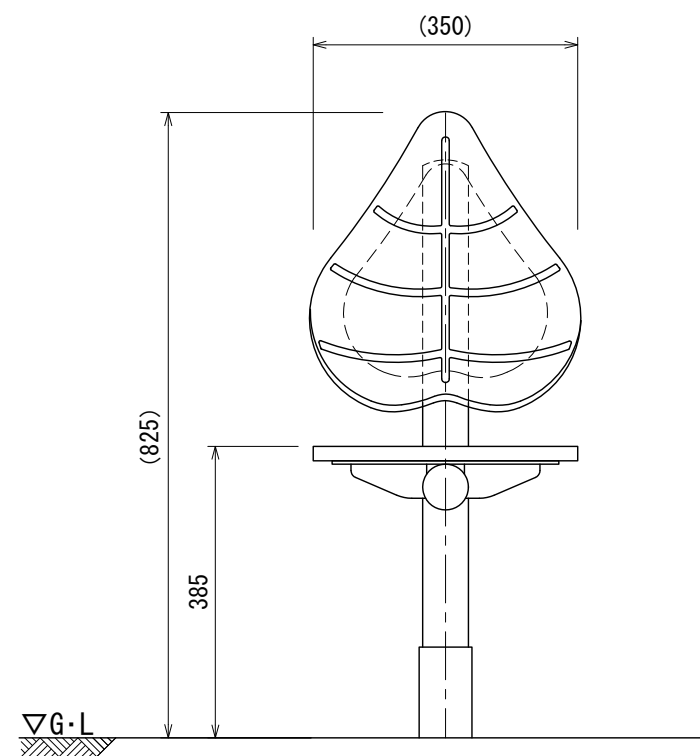
立面図
