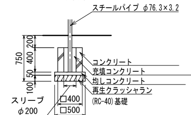
D'1基礎詳細図
