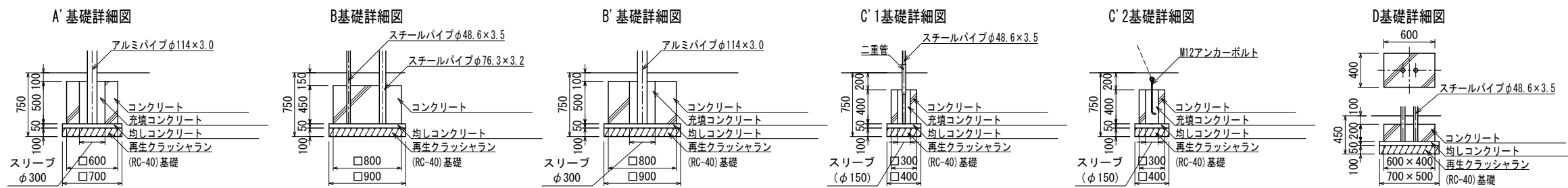
基礎詳細図 S=1:30 (A1) S=1:60 (A3)
