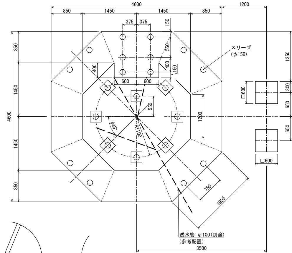
基礎伏図
