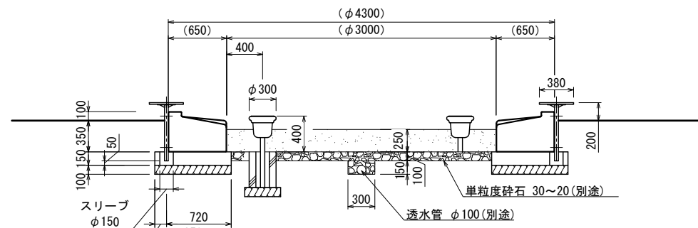
A-A' 断面図
