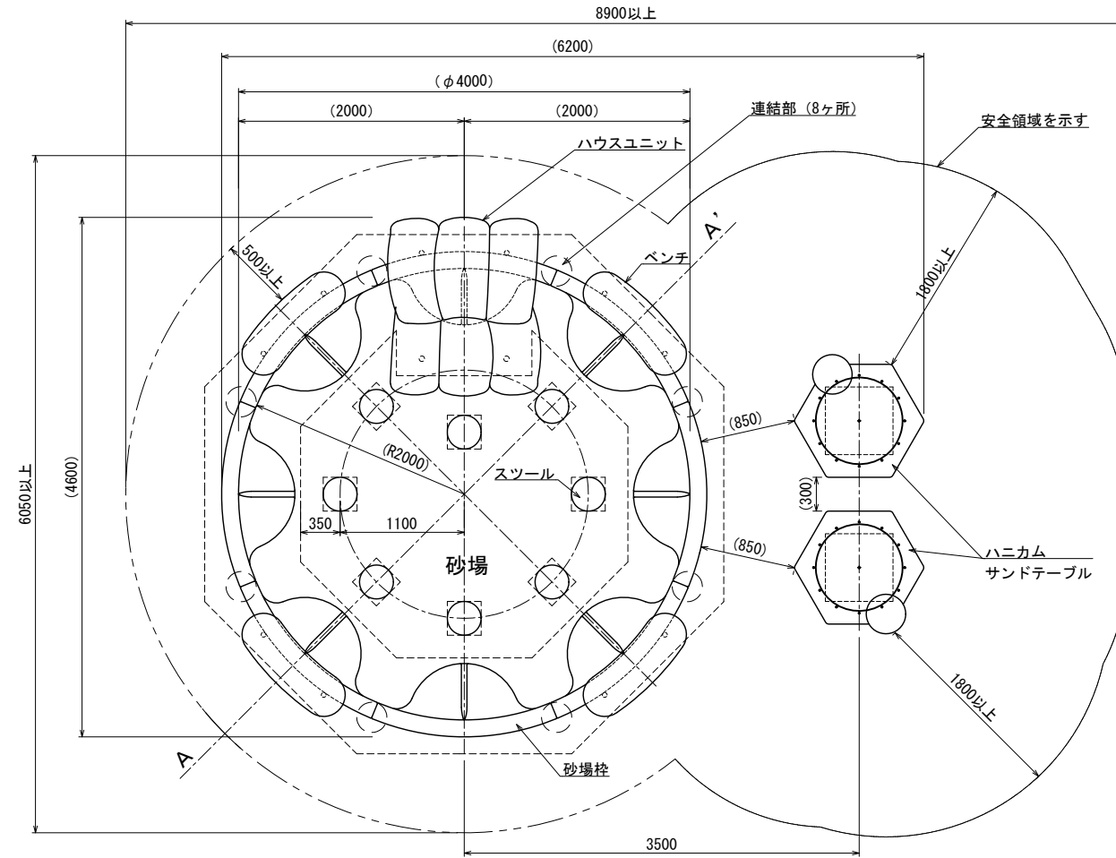
平面図
