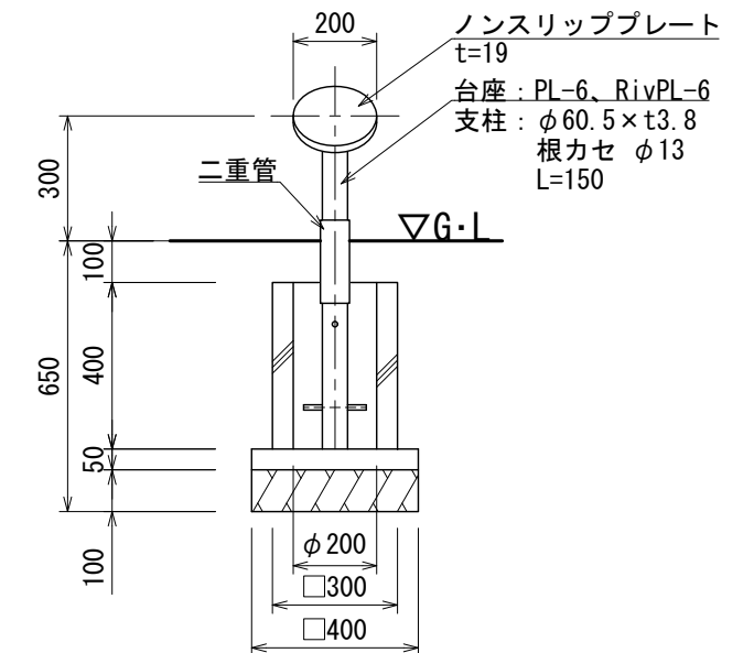
アキレスストレッチャー 詳細図
