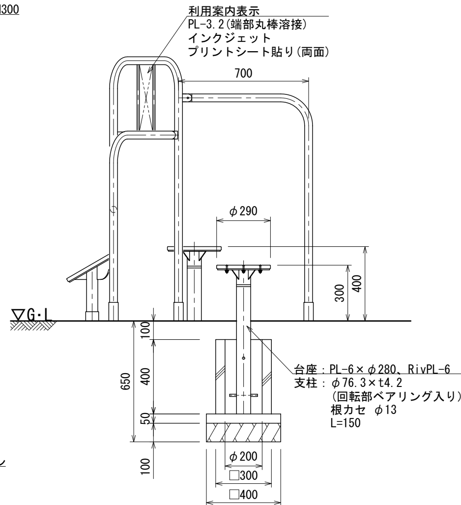
側面図
