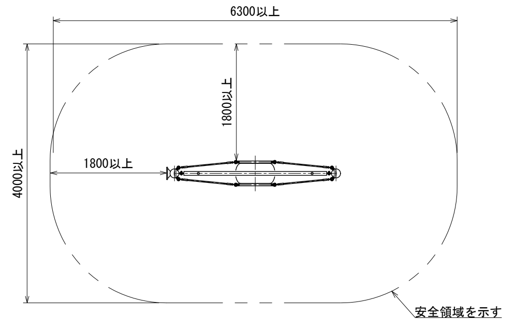
安全領域図 S=1:60
