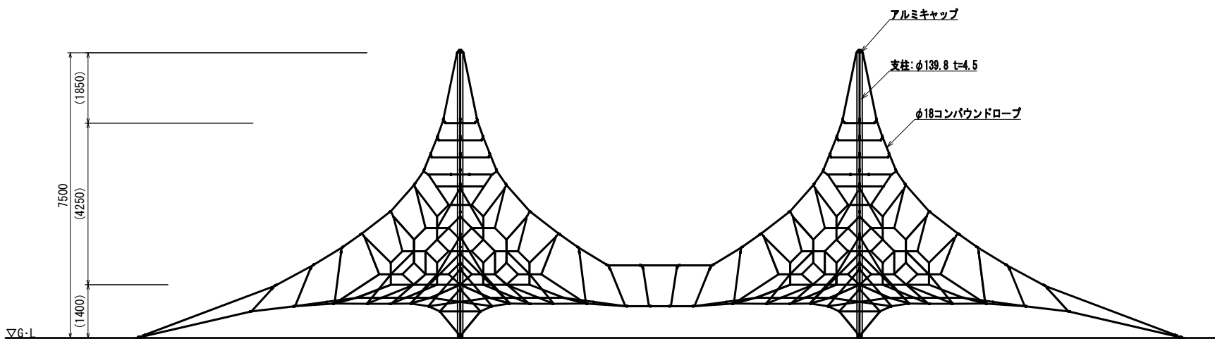
立面図
