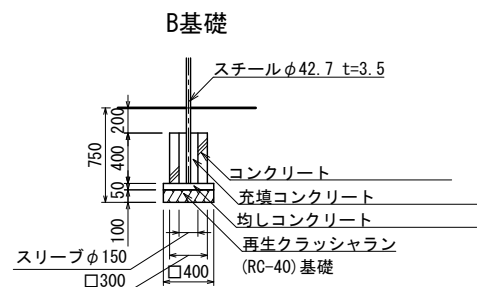
B基礎
