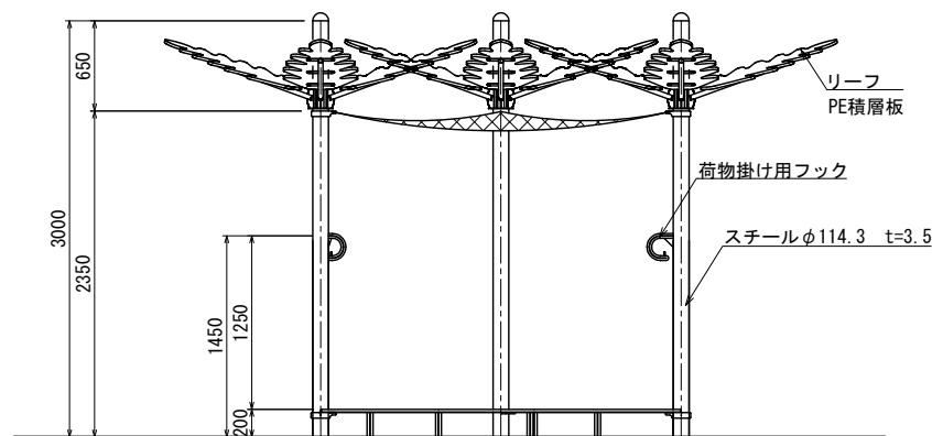
立面図
