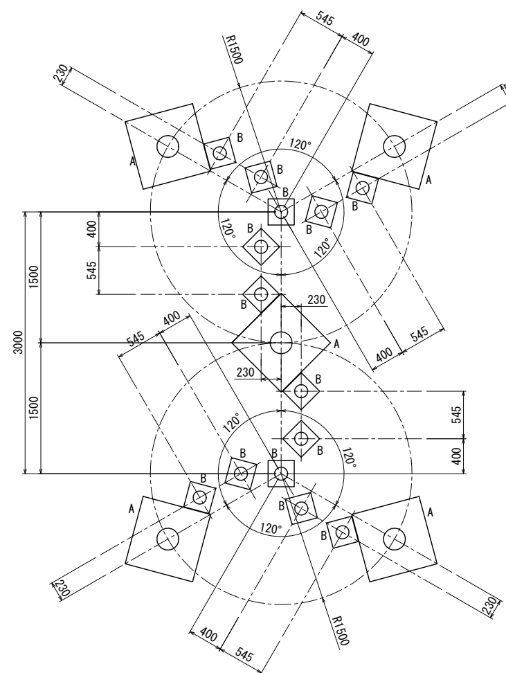
基礎伏図
