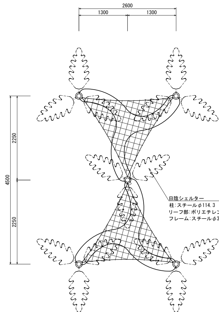
平面図
