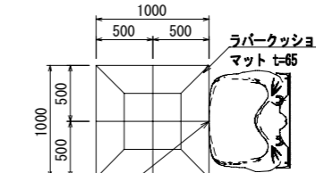
スライダー先端とマットの 中央部の端を合わせる事。
