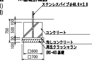
A1基礎詳細図
