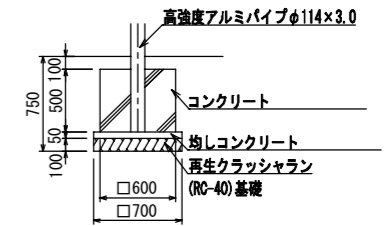
A2基礎詳細図
