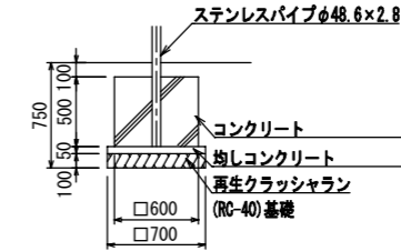
A1基礎詳細図
