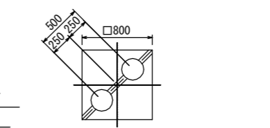
B'2基礎詳細図
