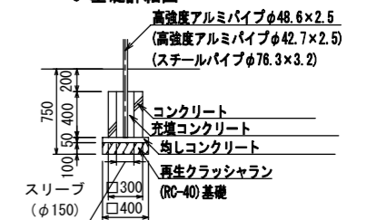
C'基礎詳細図
