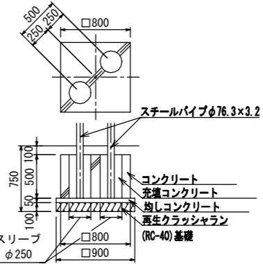
B'2基礎詳細図
