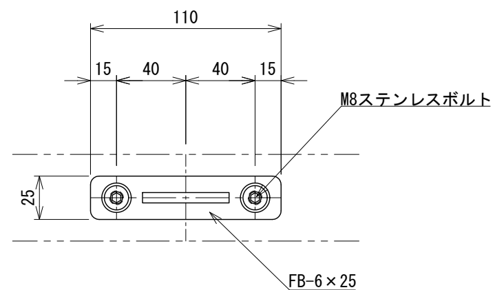
取付プレート詳細図
