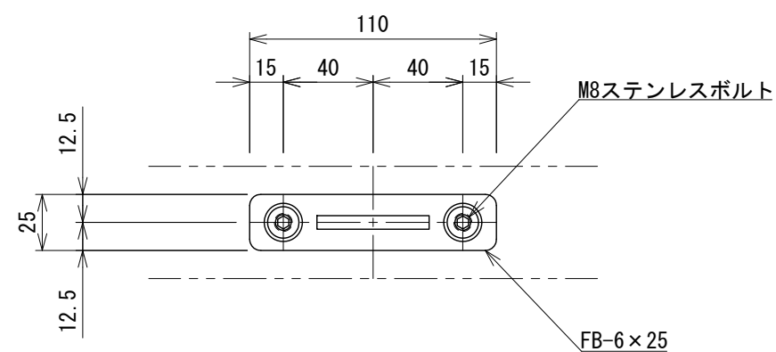
取付プレート詳細図
