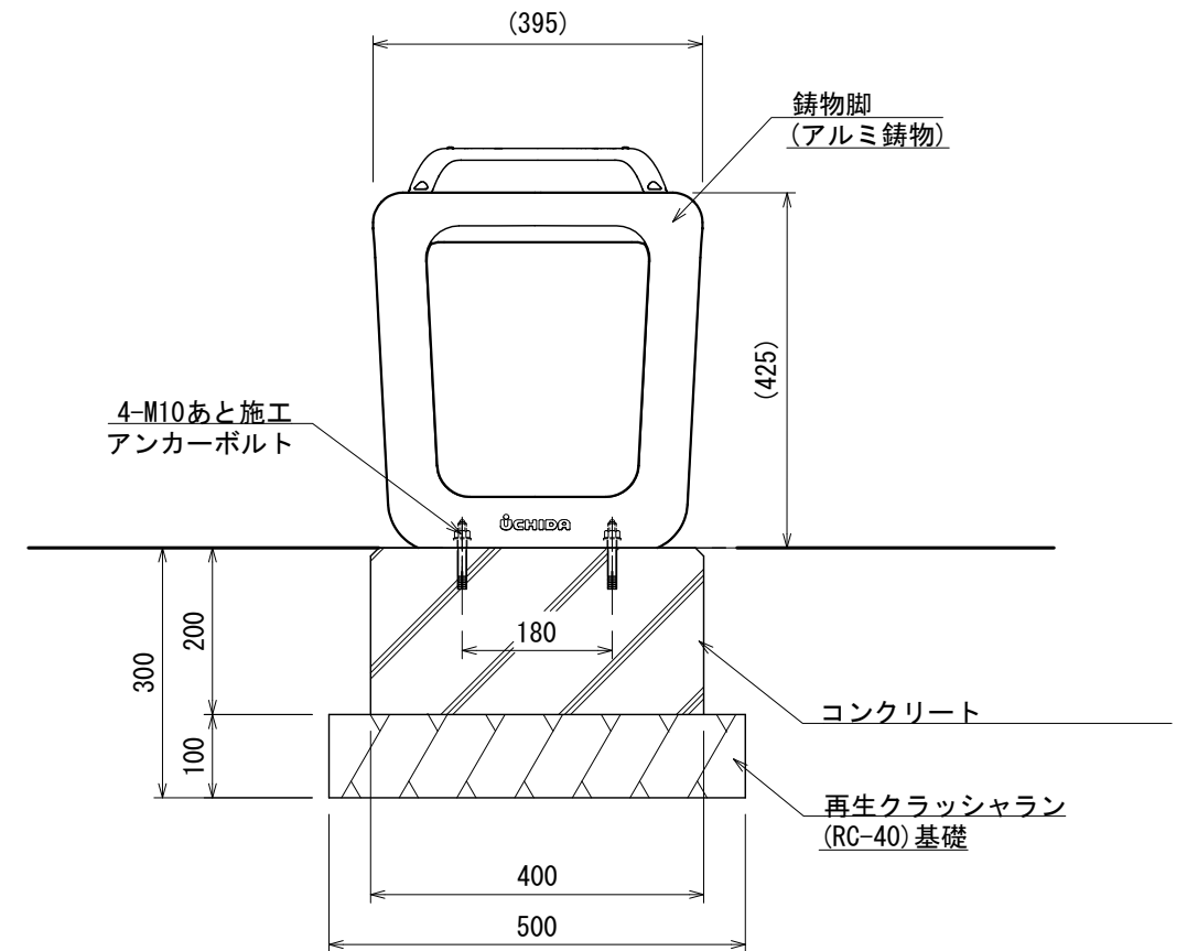
側面図
