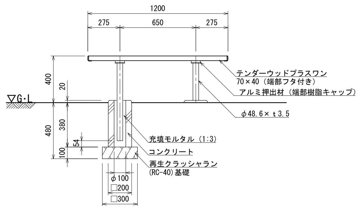
立面図
