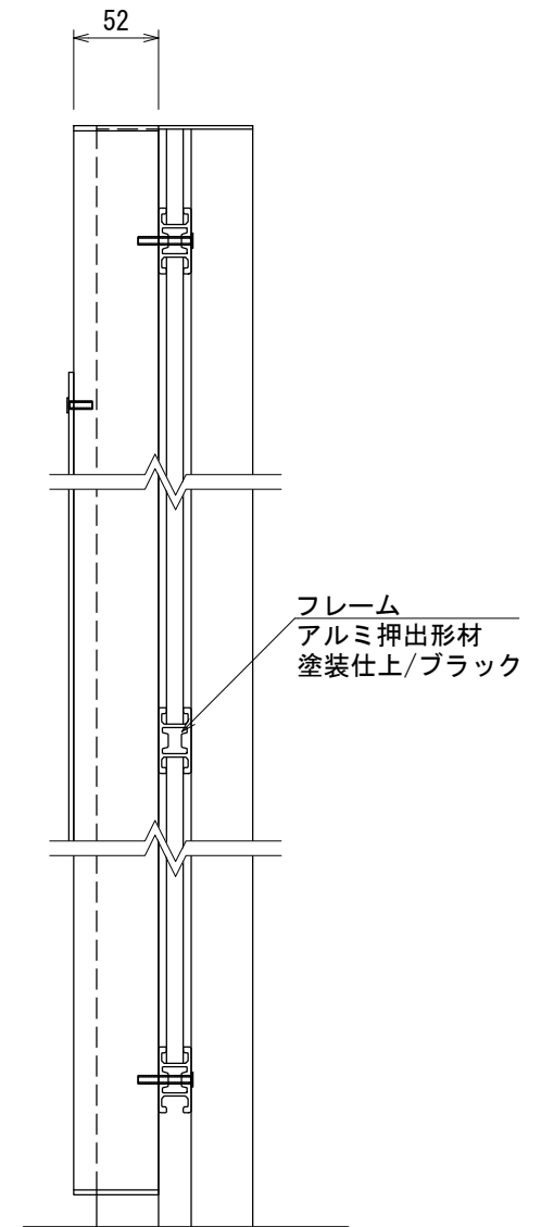
側面図 S=1:5
