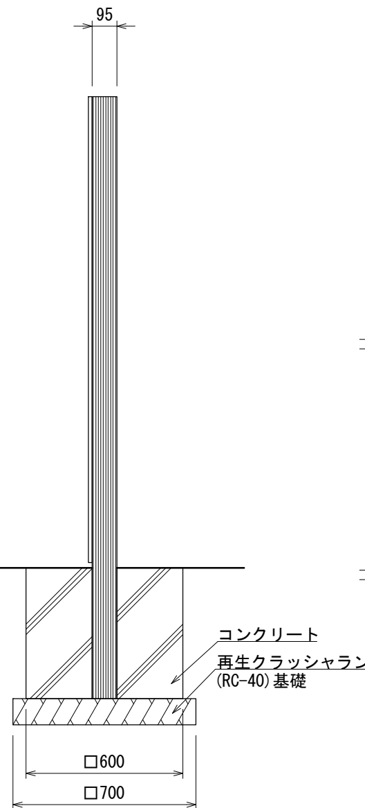
側面図
