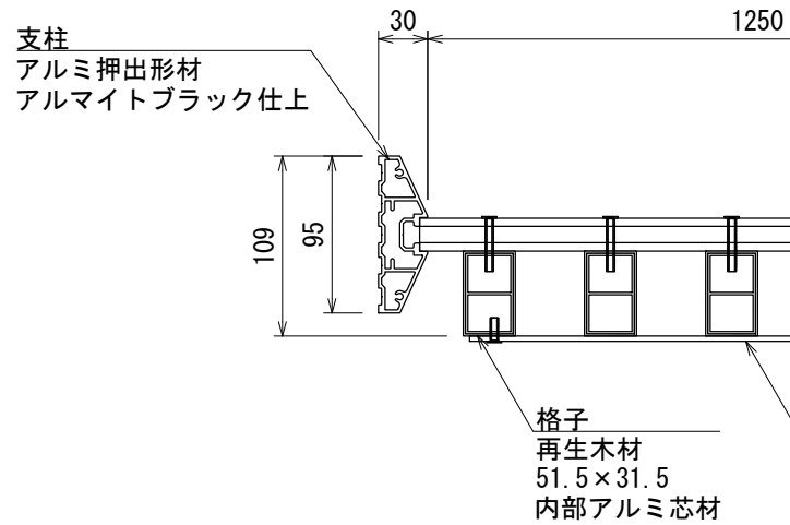
平面図 S=1:5
