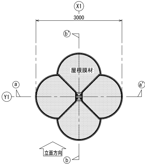
屋根伏図
