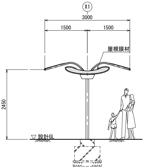
立面図
