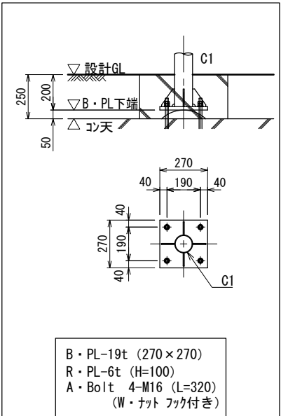
柱脚詳細図 S=1:30 (A1 S=1:15)
