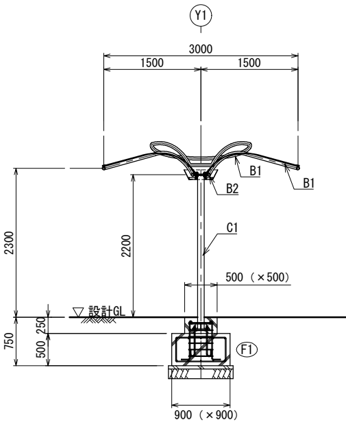
b-b' 断面図
