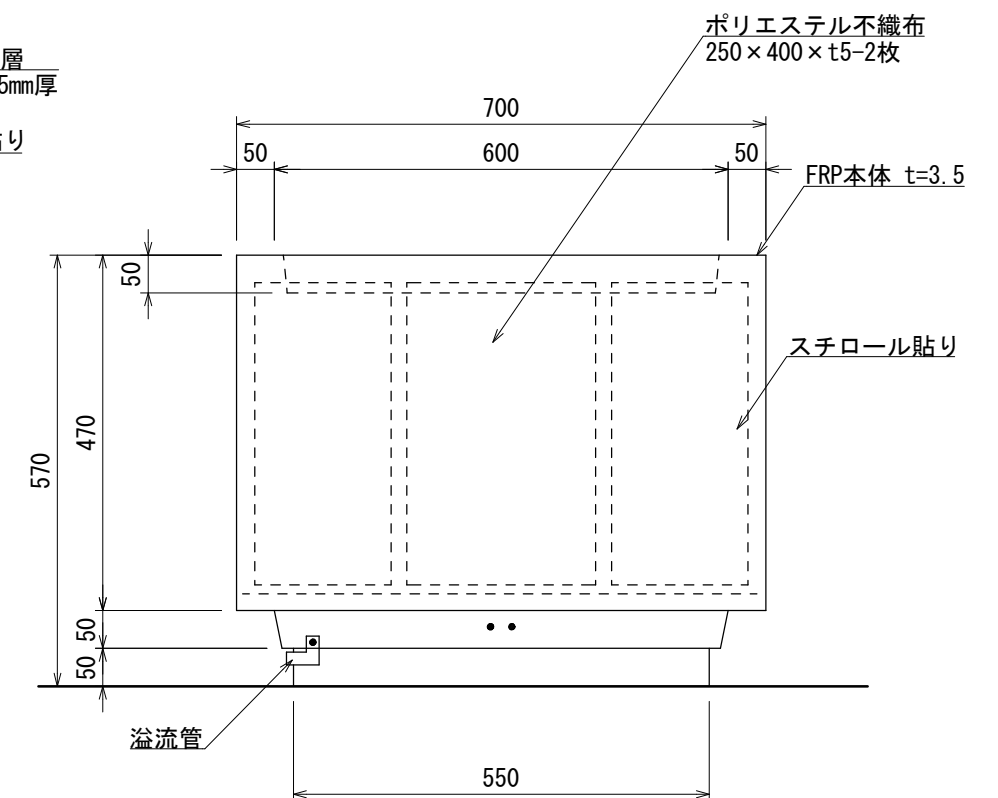
側面図
