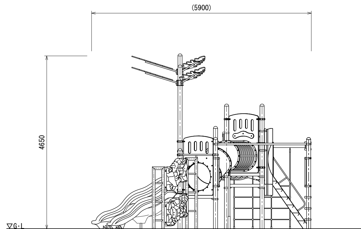
B立面図
