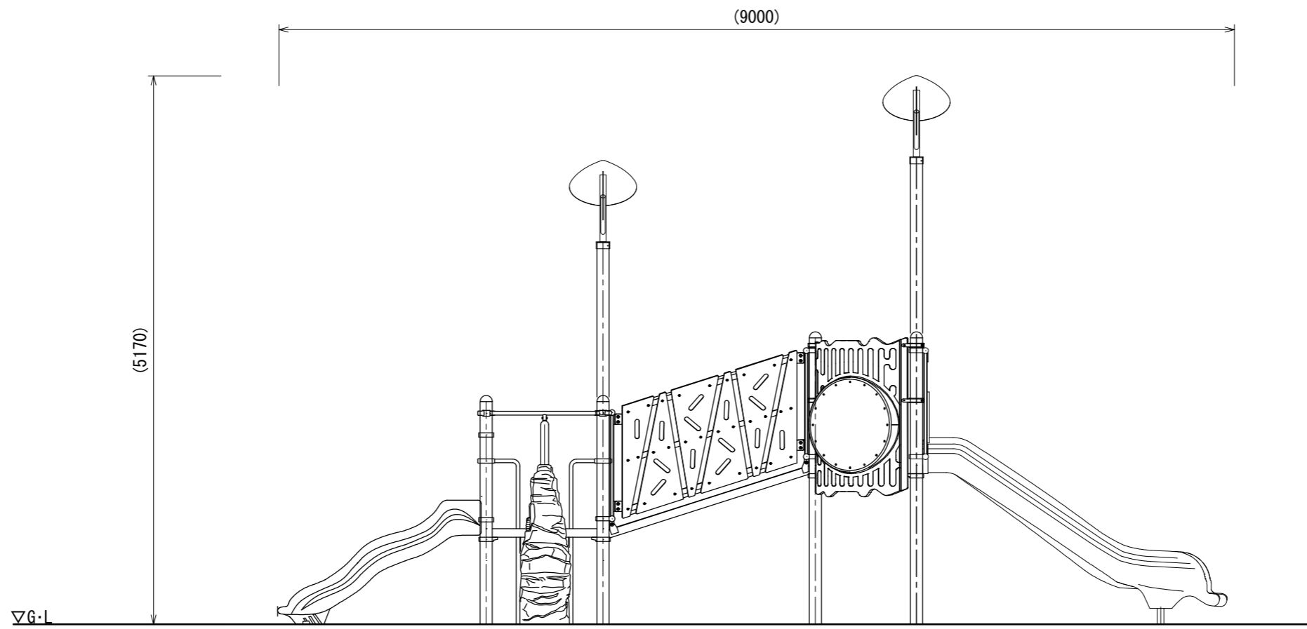
A立面図
