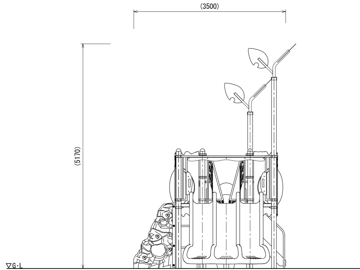
B立面図
