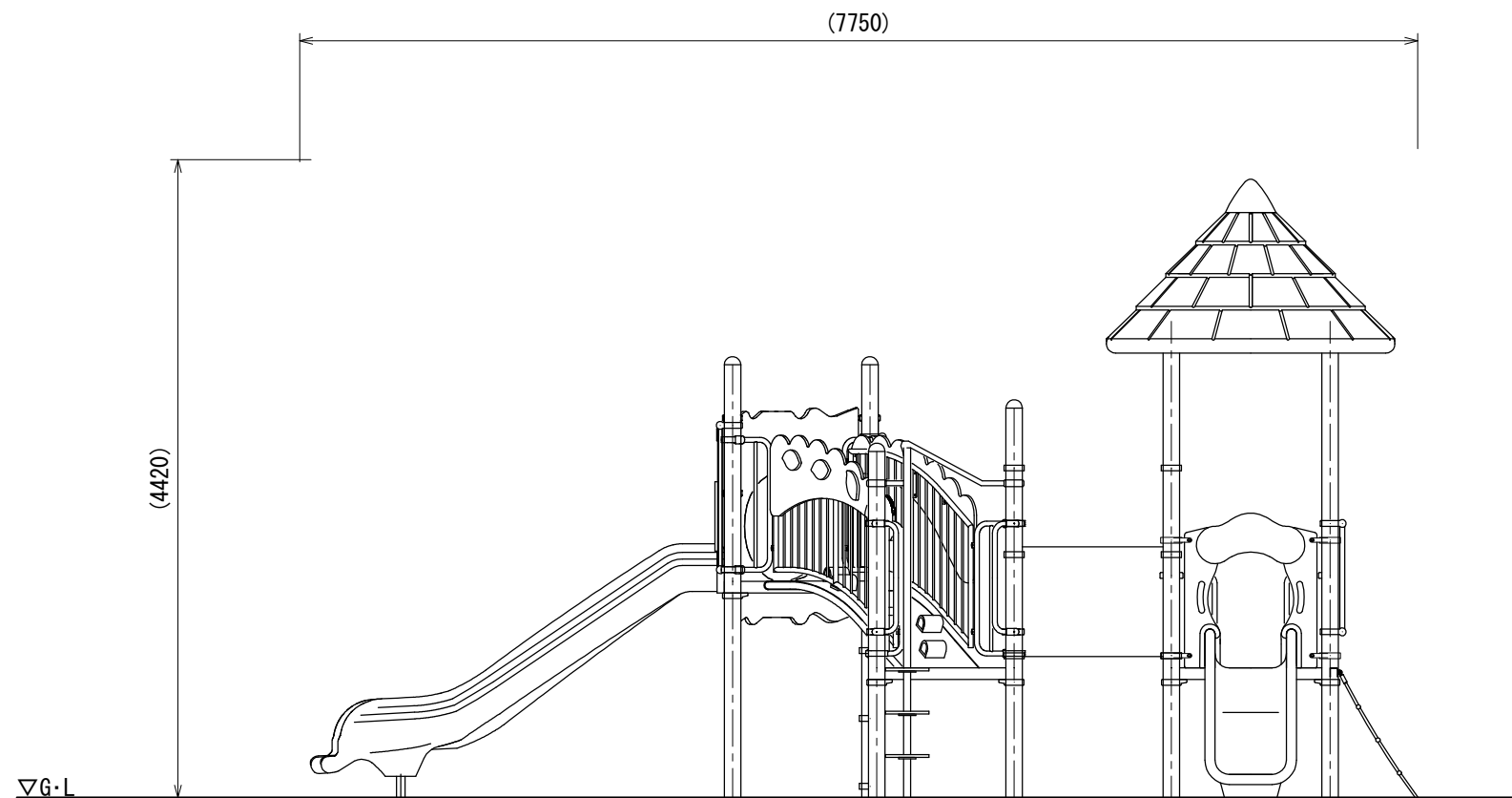
B立面図
