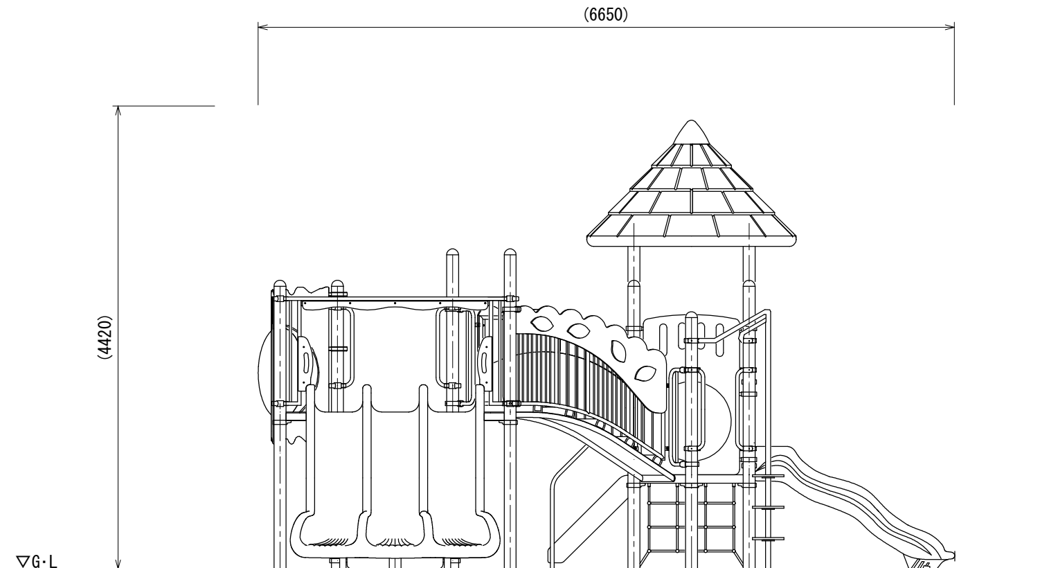
A立面図
