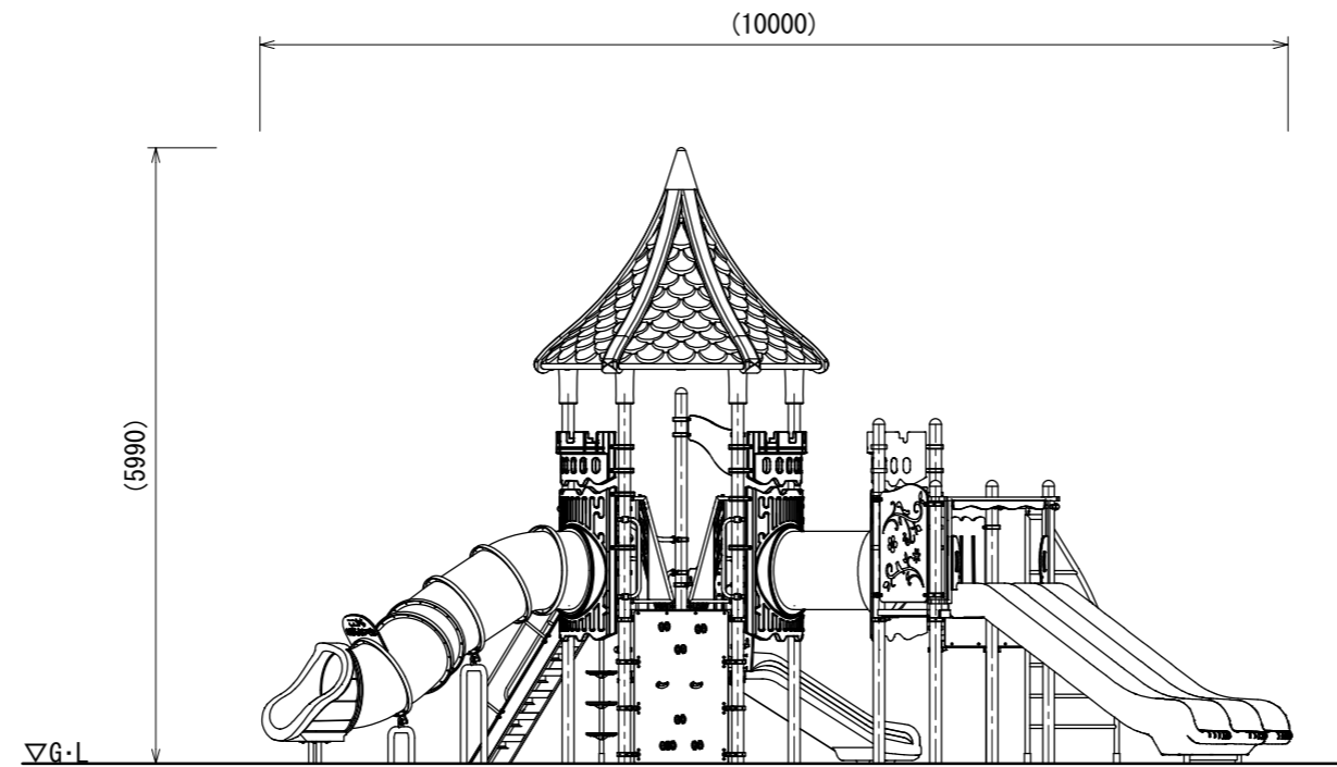
A立面図
