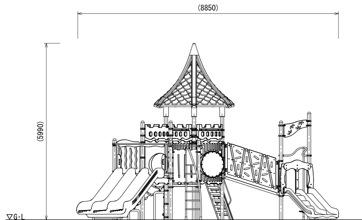
B立面図
